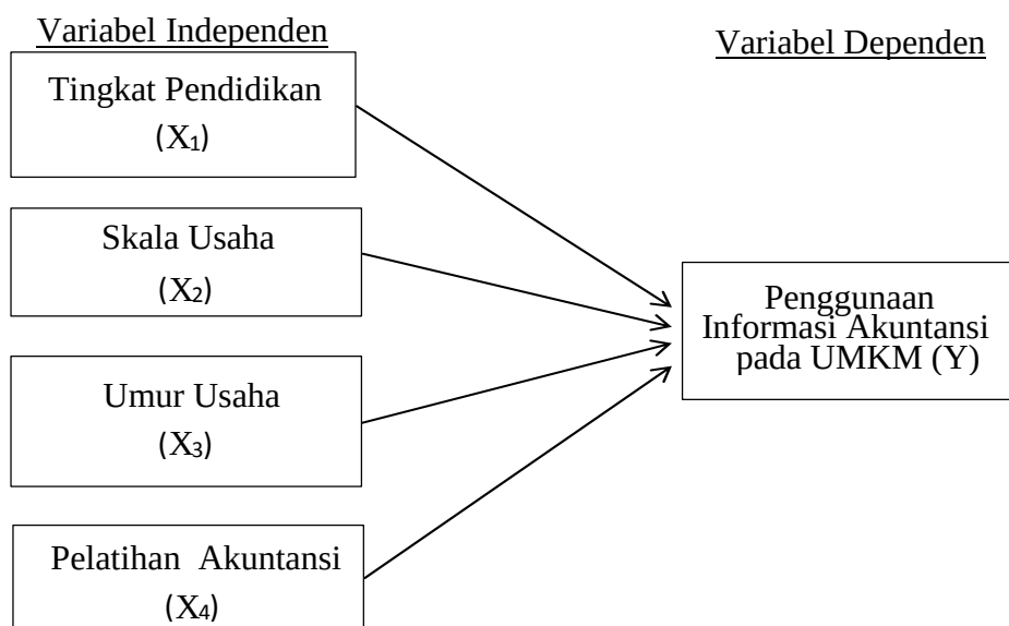
Gambar 1 Kerangka Pemikiran
