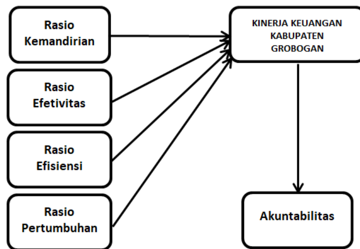
Gambar 2. 1 kerangka berpikir
